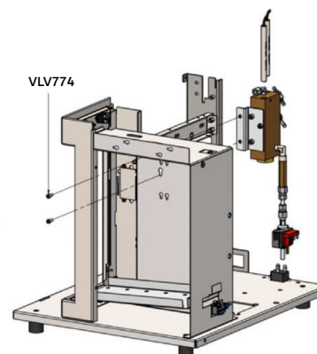
Attrezzatura per macchina CAFFÈ VAPORE Equipment for COFFEE STEAM machine Équipement pour machine CAFÉ VAPEUR
