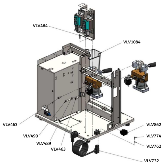
Attrezzatura per macchina CAFFÈ VAPORE Equipment for COFFEE STEAM machine Équipement pour machine CAFÉ VAPEUR
