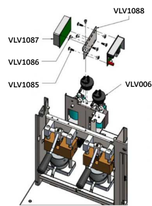
Attrezzatura per macchina VOLUMETRICA Equipment for volumetric machine Équipement pour machine volumétrique
