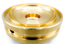
MG027 Porta pastiglia per cialda Ø38 in ottone Brass Ø38 pad holder for pod
